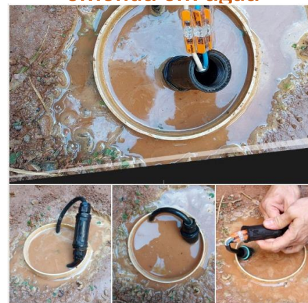
Cabo + conector de emenda em água
